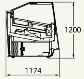
Perfettol冰淇淋柜CAD尺寸图
