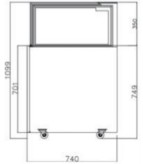
精品柜CAD尺寸图
