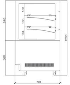
量子款蛋糕柜CAD尺寸图
