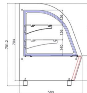
罗森款台式柜CAD尺寸图
