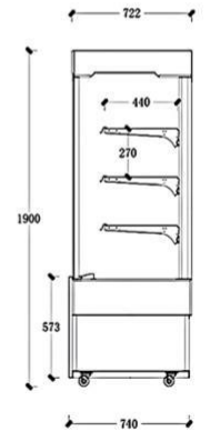
立式蛋糕柜CAD尺寸图
