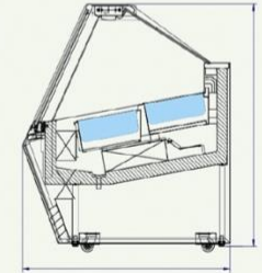
Control冰淇淋柜CAD尺寸图
