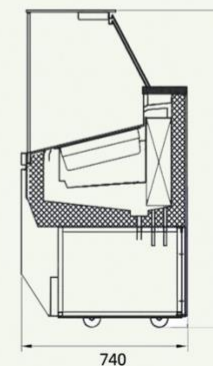
Bonjour 冰淇淋柜CAD尺寸图
