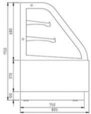
双弧柜CAD尺寸图
