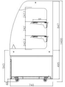
矮立风柜CAD尺寸图
