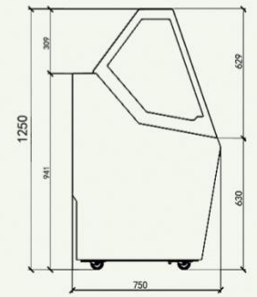
Shero冰淇淋柜CAD尺寸图
