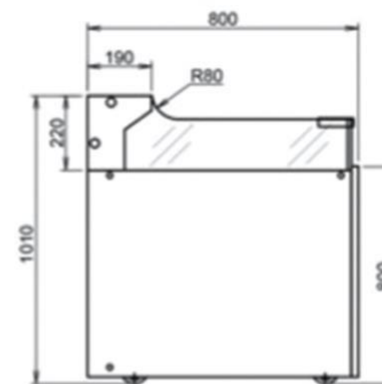
生鲜柜CAD尺寸图
