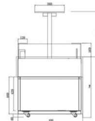
三明治柜CAD尺寸图
