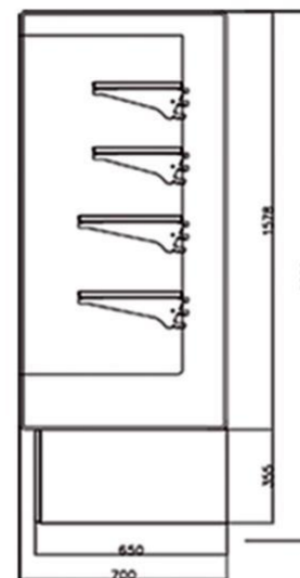
便利店款风幕柜CAD尺寸图 (异形定制)
