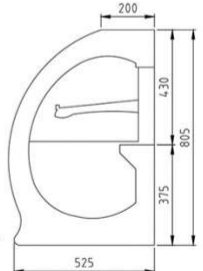
红弧柜CAD尺寸图
