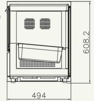
ELFI3冰淇淋柜CAD尺寸图
