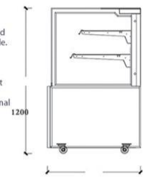
西点柜CAD尺寸图
