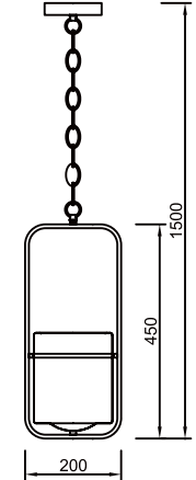
1820 Pendant lamp Matt black E27 Max. 10W
