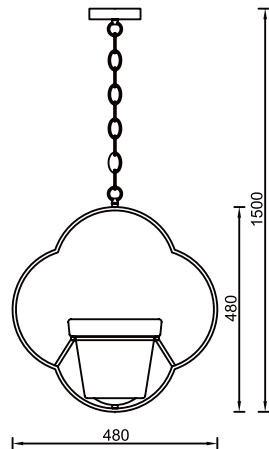
1812 Pendant lamp Matt black E27 Max. 10W
